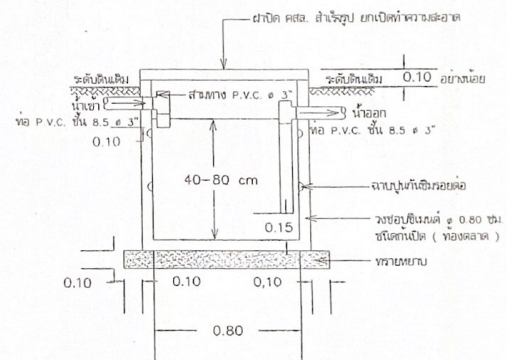
รูปตัดถังตกไขมัน
