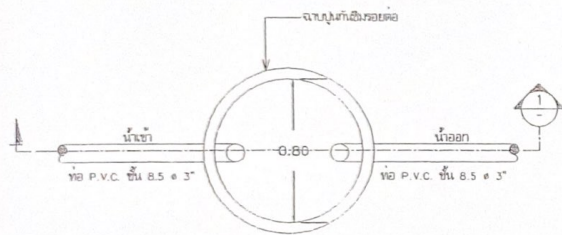
แปลนถังตกไขมัน
